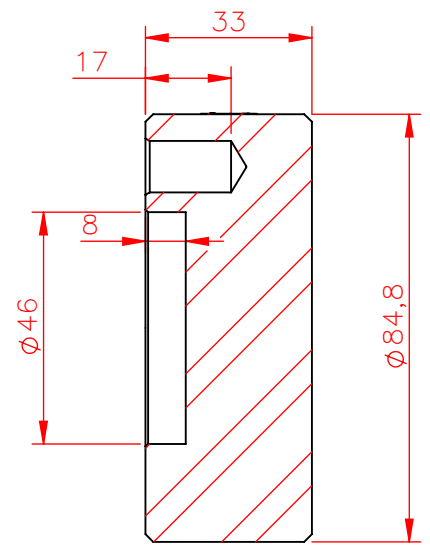
SEÇÃO B-B ESCALA 1 : 1.5
